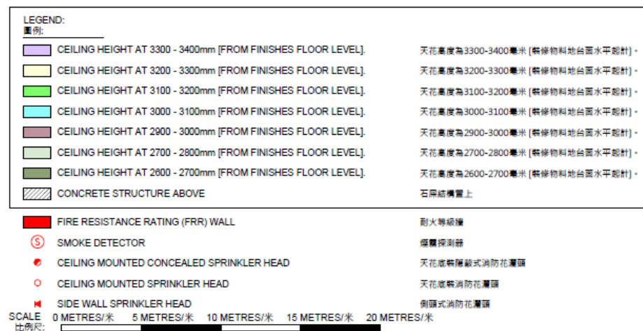
Marina Tower 2 12/F Floor Plan 漾景閣第2座 12樓平面圖
