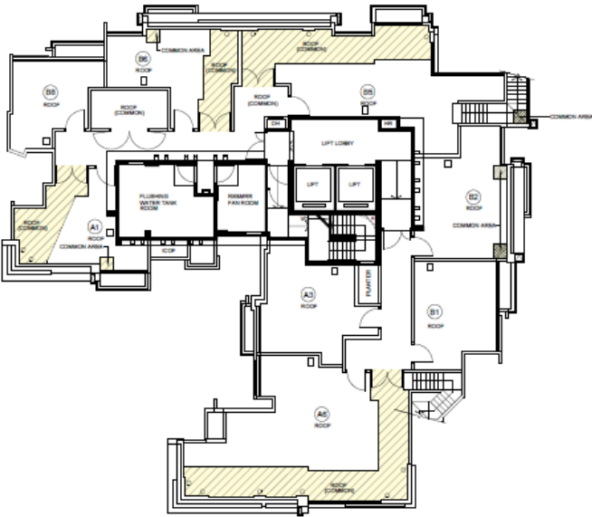
MARINA TOWER 2 ROOF FLOOR PLAN 漾景閣第2座 天台平面圖
